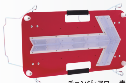
チェンジ・アロー 青 (赤地/白矢印 青LED)
