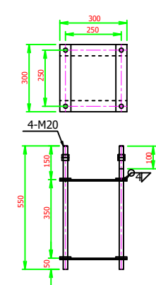
アンカーボルト詳細図
