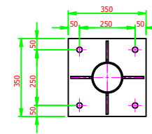
ベースプレート詳細図
