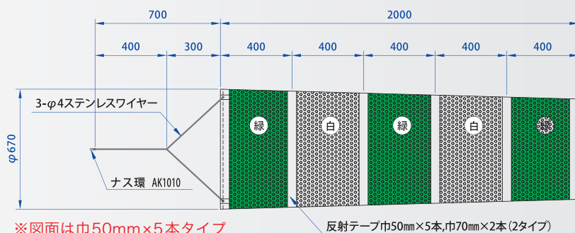
連結金具 AK1010詳細図
